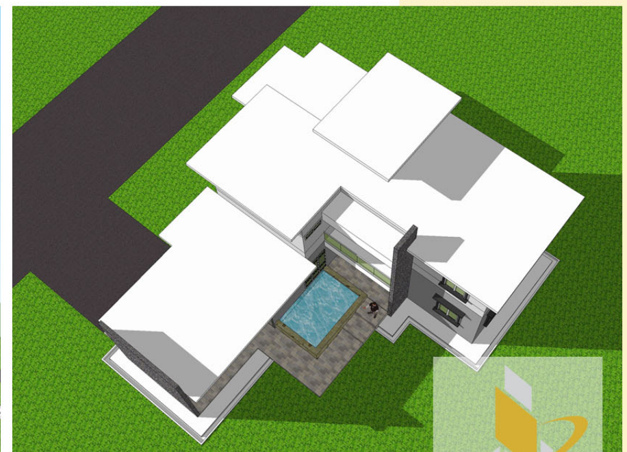
DESIGN D215 Banglo 2 Tingkat - 6 bilik/3 bilik air 2987kaki persegi
